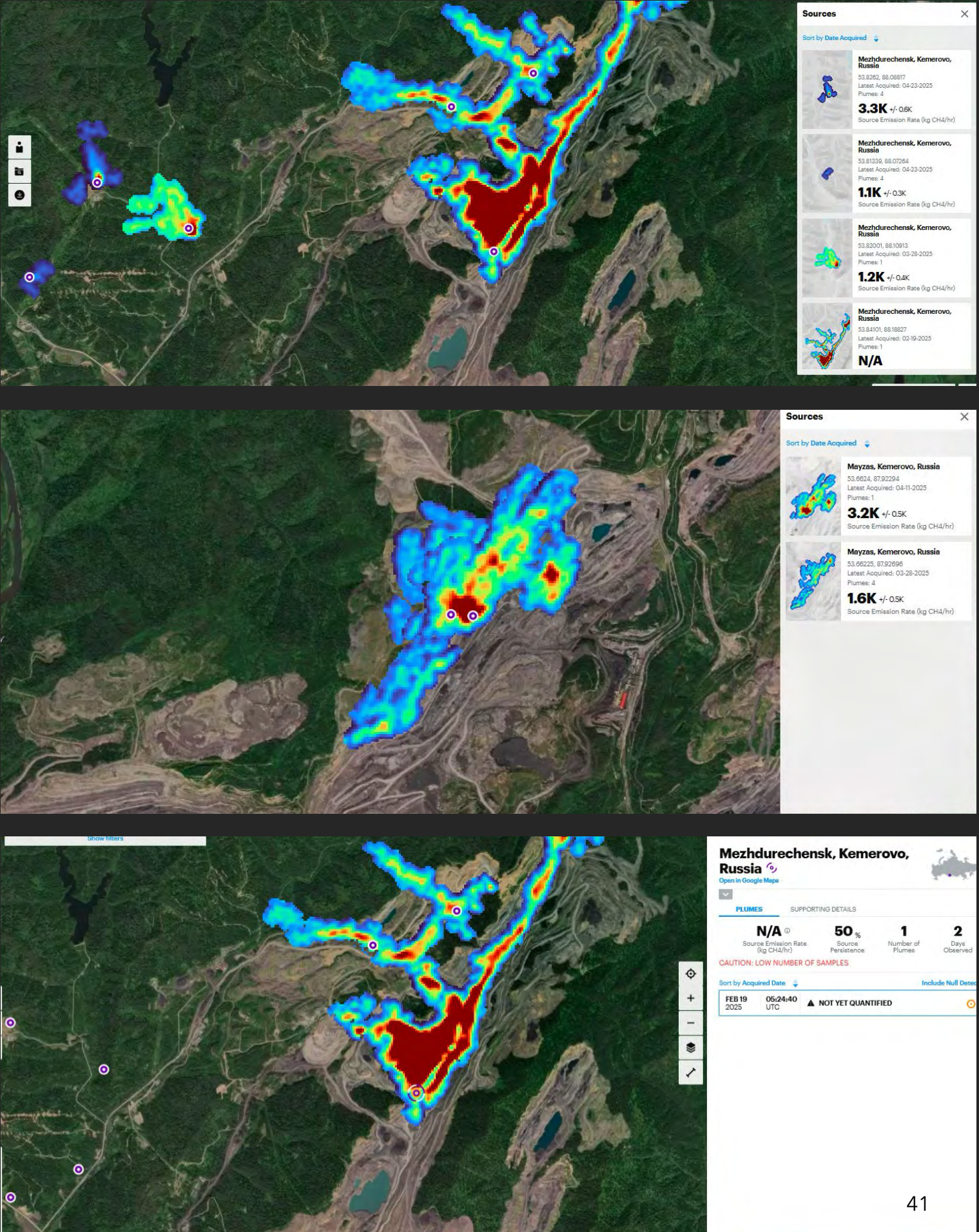
Рис 7. Некоторые случаи сверхвыбросов метана на угольных предприятиях Кузбасса
